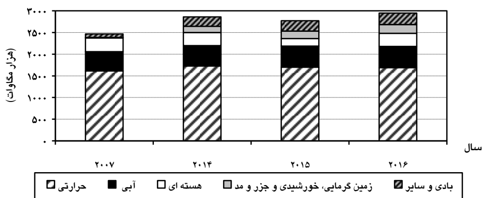
نمودار (۲-۱۷): ظرفیت نصب نیروگاه‌های برق کشورهای OECD در سال‌های ۲۰۰۷ و ۲۰۱۴-۱۶
