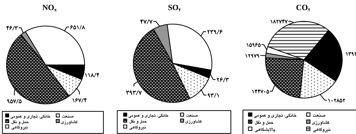
نمودار (۲۶-۱): میزان انتشار SO ۲ ، CO ۲ و NO x از بخش‌های مختلف انرژی در سال ۱۳۹۶ (هزار تن)
